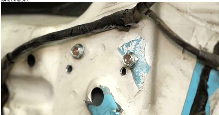
22 Kiristä ikkunannostimen mekanismin kiinnikkeet. Käytä 10 mm:n hylsyä. Käytä momenttiavainta. Kiristysmomentti: 8 N·m.
