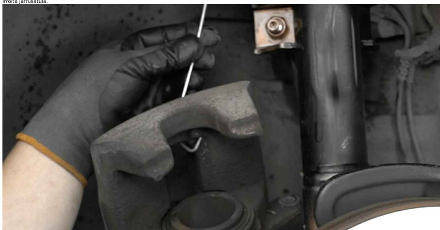
Vaihto: jarrupalojen kulumisen ilmaisin - MERCEDES-BENZ E-sarja Coupe (C207). Vinkki:
