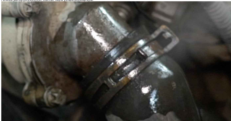
16 Löysää jäähdytysnesteletkujen kiristimet. Käytä clic-R-letkupihtejä.
